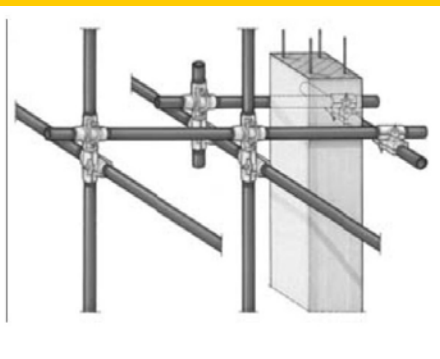
Anclaje por corbata, realizado sobre pilar
